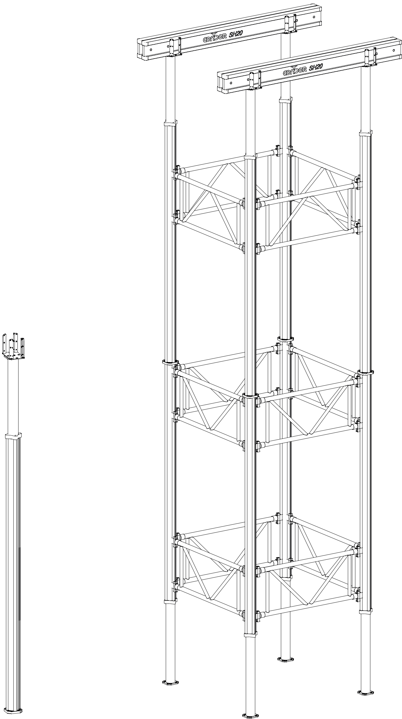
Puntello ALUCP
